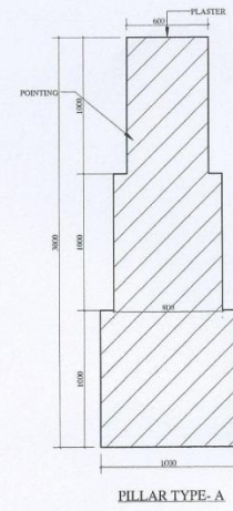
PILLAR TYPE-A
