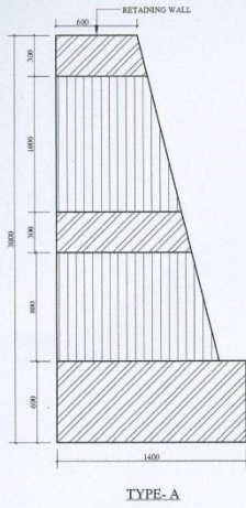
TYPE-A
